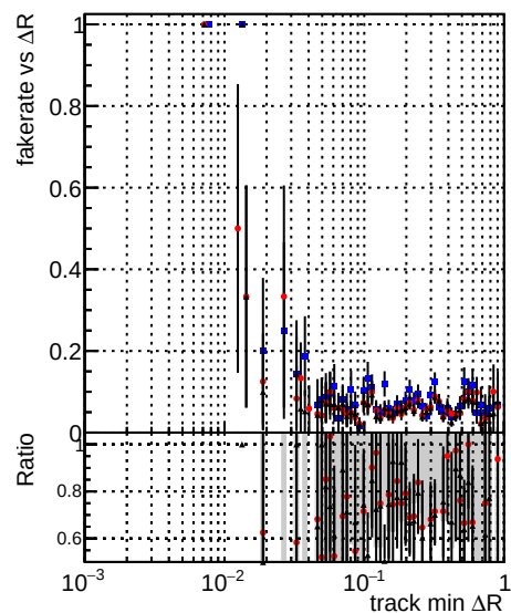
—●— DQMstep3_SoftQCD_CKF —●— DQMstep3_SoftQCD_default —●— DQMstep3_SoftQCD_ckfPileLess
