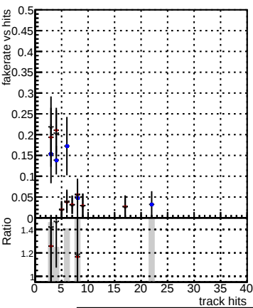
Fake rate vs hit —●— DQMstep3_SoftQCD_CKF —■— DQMstep3_SoftQCD_default —●— DQMstep3_SoftQCD_ckfPixelLess
