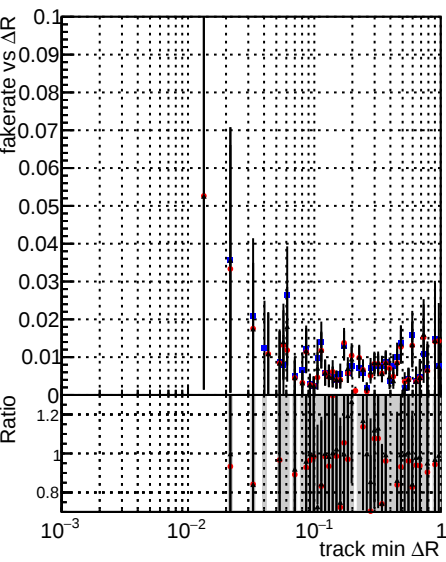
Fake rate vs \Delta R(\text{track, jet}) DOMstep3_SoftQCD_CKF DOMstep3_SoftQCD_default DOMstep3_SoftQCD_ckfPixelLess
