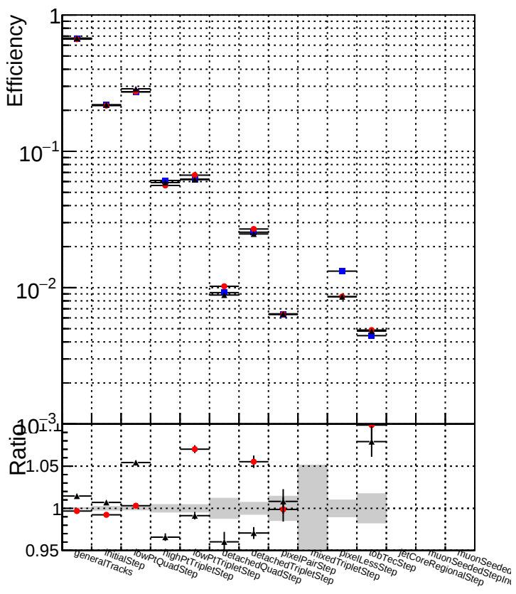
DQMstep3_SoftQCD_CKF DQMstep3_SoftQCD_default DQMstep3_SoftQCD_defaultNEWT
