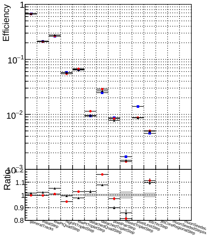
DQMstep3_SoftQCD_CKF DQMstep3_SoftQCD_default DQMstep3_SoftQCD_defaultNEWT
