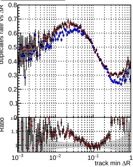
Legend: —•— DOMstep3 SoftQCD CKF —•— DOMstep3 SoftQCD default —•— DOMstep3 SoftQCD defaultNEWT
