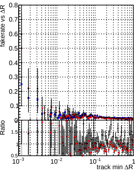
Legend: DQMstep3_SoftQCD_CKF (blue), DQMstep3_SoftQCD_default (red), DQMstep3_SoftQCD_defaultNEWT (black)
