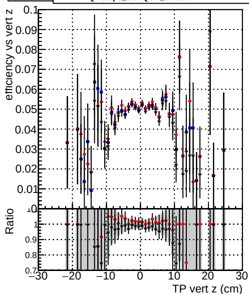
Efficiency vs vert z ● DQMstep3_SoftQCD_CKF ● DQMstep3_SoftQCD_default ● DQMstep3_SoftQCD_defaultNEWT
