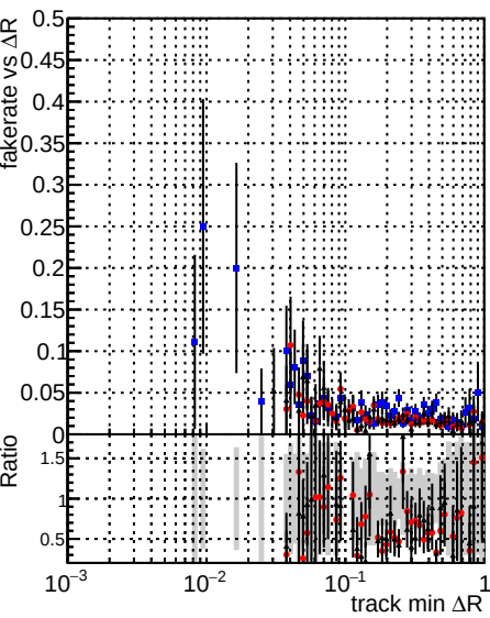
DOMstep3 SoftQCD CKF DOMstep3 SoftQCD default DOMstep3 SoftQCD defaultNEWT
