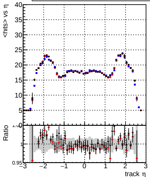
mean hit — DQMstep3_SoftQCD_CKF — DQMstep3_SoftQCD_default — DQMstep3_SoftQCD_defaultNEWT
