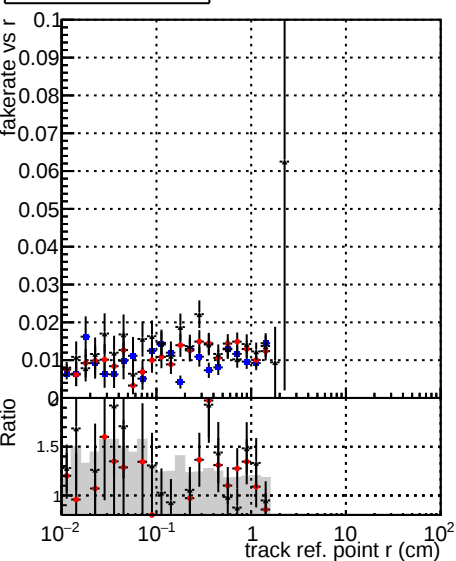
Fake rate vs verpos DOMstep3_SoftQCD_CKF DOMstep3_SoftQCD_default DOMstep3_SoftQCD_defaultNEWT
