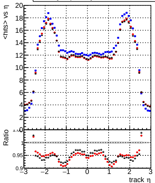
— DQMstep3_SoftQCD_CKF — DQMstep3_SoftQCD_default — DQMstep3_SoftQCD_defaultNEWT mean hit
