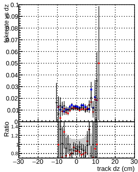
Fake rate vs dz DOMstep3 SoftOCD-CKF DOMstep3 SoftOCD-default DOMstep3 SoftOCD-defaultNEWT
