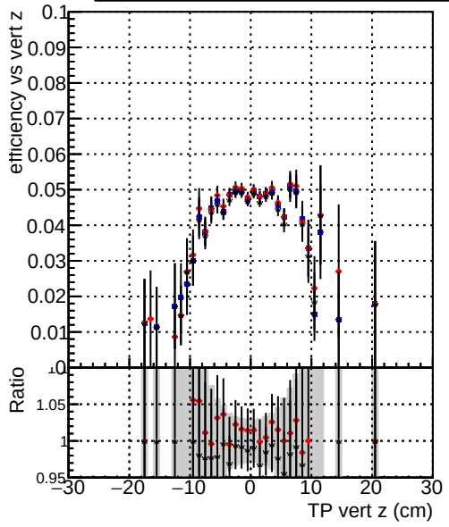
Efficiency vs. TP vert z (cm) — DQMstep3_SoftQCD_CKF — DQMstep3_SoftQCD_default — DQMstep3_SoftQCD_defaultNEWT
