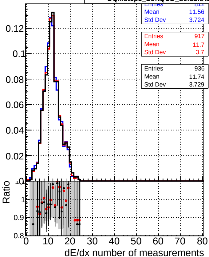
—■— DQMstep3_SoftQCD_CKF —●— DQMstep3_SoftQCD_default —▲— DQMstep3_SoftQCD_defaultNEWT
