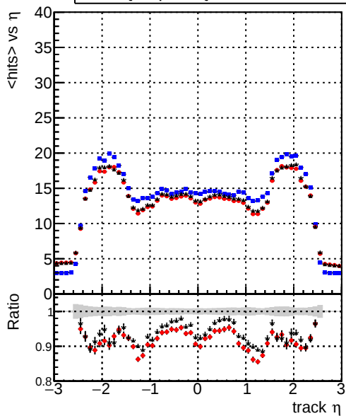
— DQMstep3_SoftQCD_CKF — DQMstep3_SoftQCD_default — DQMstep3_SoftQCD_defaultNEWT
