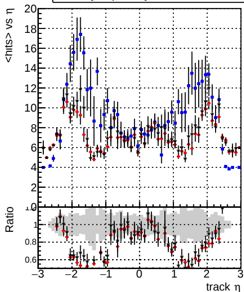
mean hits vs \eta — DQMstep3_SoftQCD_CKF — DQMstep3_SoftQCD_default — DQMstep3_SoftQCD_defaultNEWT
