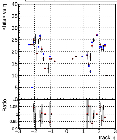
mean hits — DQMstep3_SoftQCD_CKF — DQMstep3_SoftQCD_default — DQMstep3_SoftQCD_defaultNEWT
