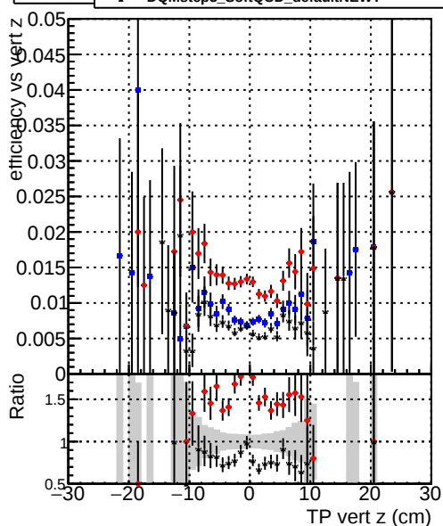
Efficiend —●— DQMstep3_SoftQCD_default —▲— DQMstep3_SoftQCD_defaultNEWT
