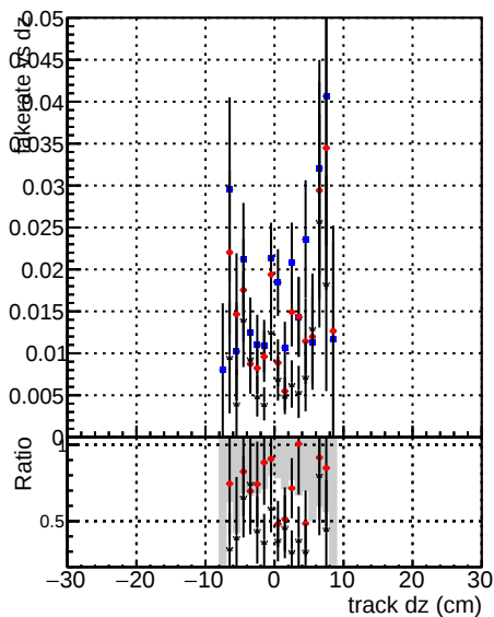
Fake rate vs dz — DOMstep3 SoftQCD CKF — DOMstep3 SoftQCD default — DOMstep3 SoftQCD defaultNEWT
