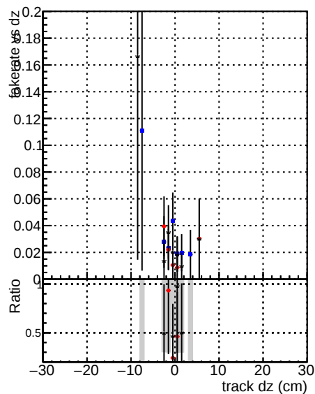
DOMstep3 SoftQCD CKF DOMstep3 SoftQCD default DOMstep3 SoftQCD NEWT
