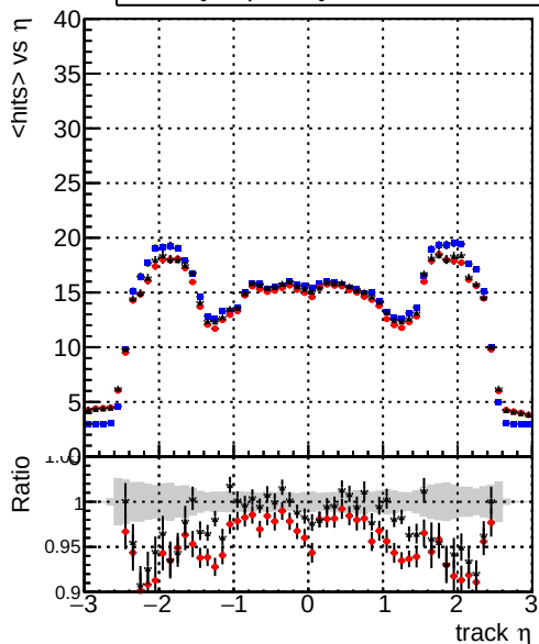
— DQMstep3_SoftQCD_CKF — DQMstep3_SoftQCD_default — DQMstep3_SoftQCD_defaultNEWT mean hit
