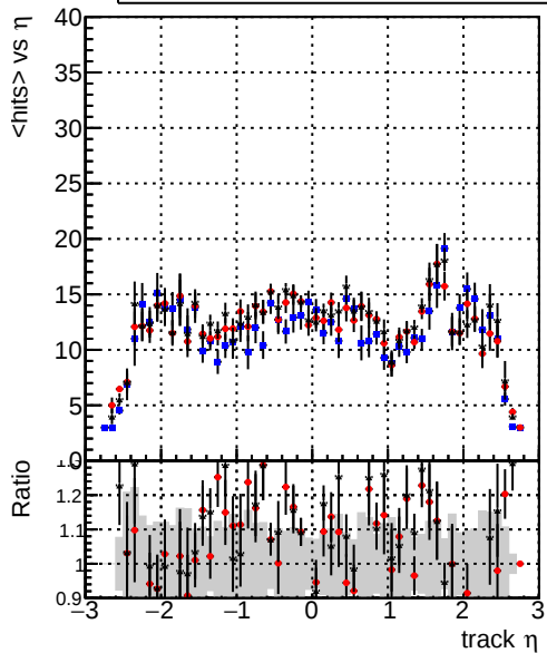
mean hit — DQMstep3_SoftQCD_CKF — DQMstep3_SoftQCD_default — DQMstep3_SoftQCD_defaultNEWT
