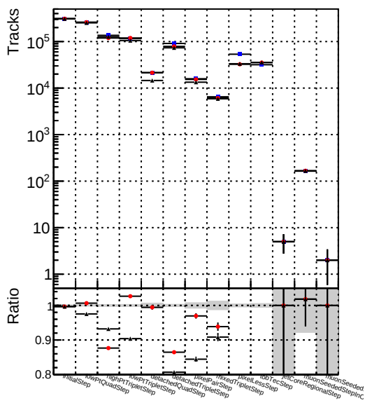
Number of tracks vs collection Legend: DQMstep3_SoftQCD_CKF (Blue) DQMstep3_SoftQCD_default (Red) DQMstep3_SoftQCD_defaultNEWT (Black)
