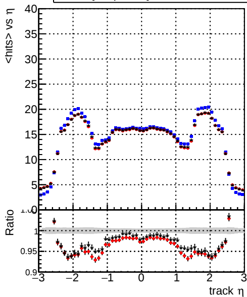
mean hits vs \eta — DQMstep3_SoftQCD_CKF — DQMstep3_SoftQCD_default — DQMstep3_SoftQCD_defaultNEWT
