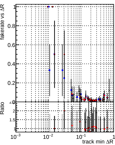
Legend: DQMstep3_SoftQCD_CKF (blue dots), DQMstep3_SoftQCD_default (red dots), DQMstep3_SoftQCD_defaultNEWT (black dots)
