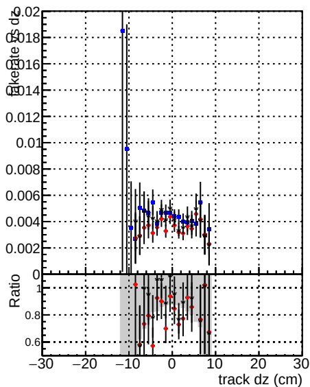
—•— DOMstep3 SoftOCD-CKF —•— DOMstep3 SoftOCD-default —•— DOMstep3 SoftOCD-defaultNEWT
