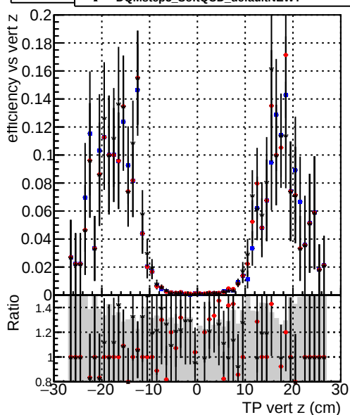
Efficiency —●— DQMstep3_SoftQCD_default —★— DQMstep3_SoftQCD_defaultNEWT
