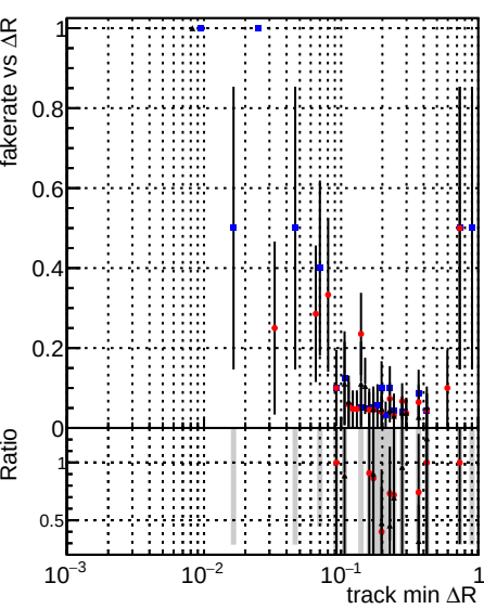
Legend: DQMstep3 SoftQCD CKF (blue squares), DQMstep3 SoftQCD default (red circles), DQMstep3 SoftQCD defaultNEWT (black circles)
