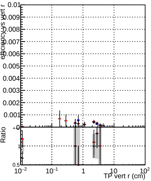
Efficiency vs vertpos DQMstep3_SoftQCD_CKF DQMstep3_SoftQCD_default DQMstep3_SoftQCD_defaultNEWT2
