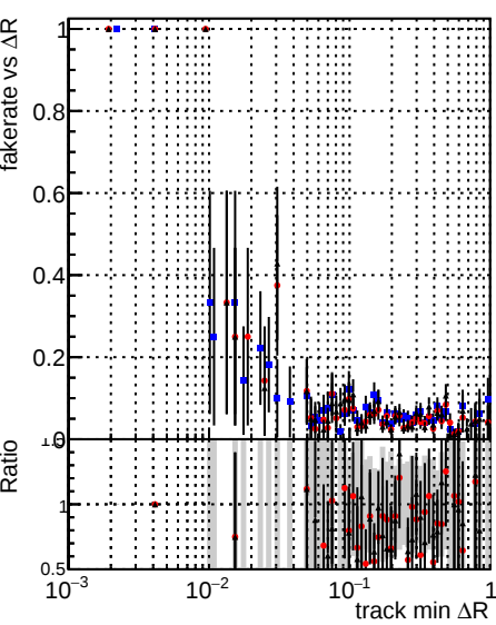
Legend: DQMstep3_SoftQCD_CKF (blue squares), DQMstep3_SoftQCD_default (red circles), DQMstep3_SoftQCD_defaultNEWT2 (black triangles)
