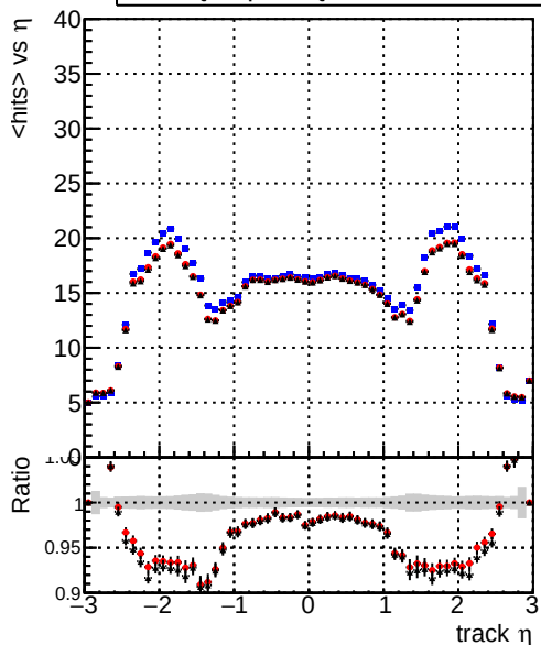
mean hits vs \eta — DQMstep3_SoftQCD_CKF — DQMstep3_SoftQCD_default — DQMstep3_SoftQCD_defaultNEWT2
