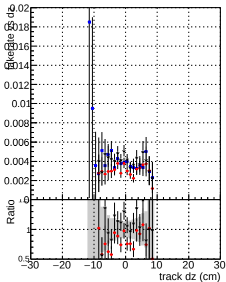
— DOMstep3 SoftQCD CKF — DOMstep3 SoftQCD default — DOMstep3 SoftQCD NEWT2
