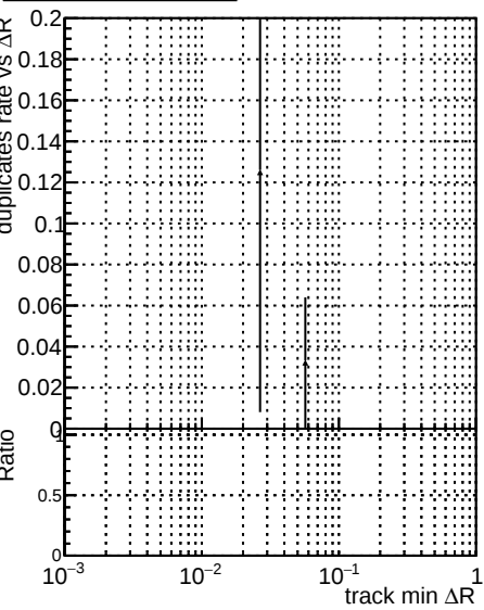
Legend: DQMstep3_SoftQCD_CKF (blue squares), DQMstep3_SoftQCD_default (red circles), DQMstep3_SoftQCD_defaultNEWT2 (black crosses)
