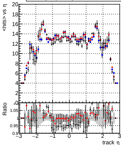
— DQMstep3_SoftQCD_CKF — DQMstep3_SoftQCD_default — DQMstep3_SoftQCD_defaultNEWT2 mean hits
