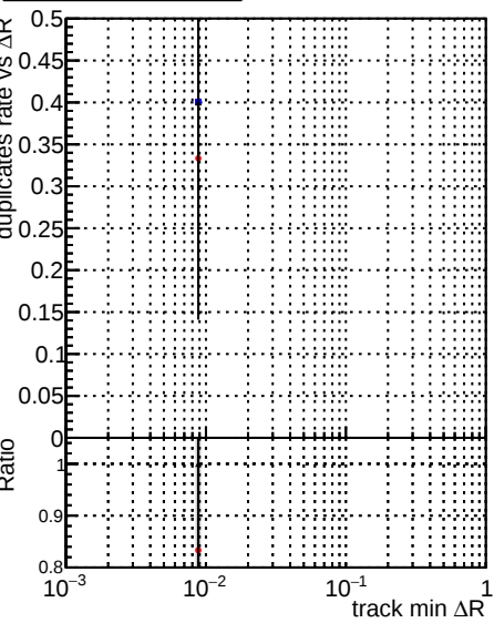
Legend: DQMstep3_SoftQCD_CKF (blue dots), DQMstep3_SoftQCD_default (red dots), DQMstep3_SoftQCD_defaultNEW2 (black dots)
