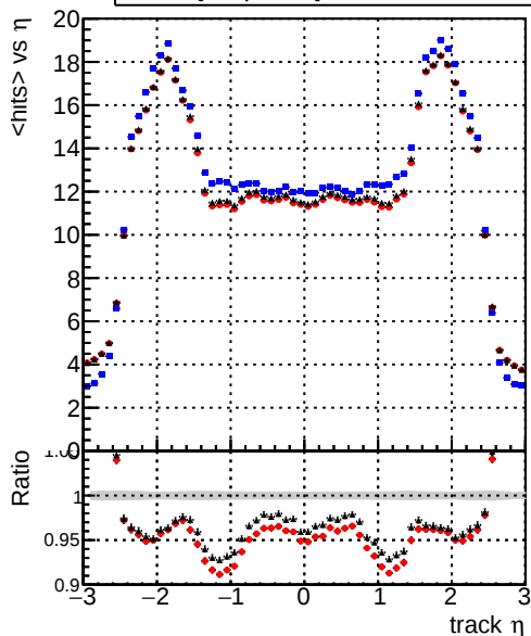
mean hit — DQMstep3_SoftQCD_CKF — DQMstep3_SoftQCD_default — DQMstep3_SoftQCD_defaultNEWT2
