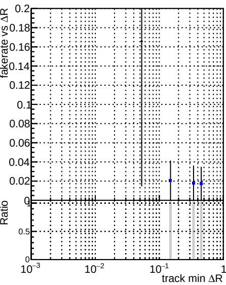
Legend: DOMstep3_SoftQCD_CKF, DOMstep3_SoftQCD_default, DOMstep3_SoftQCD_defaultNEWT2
