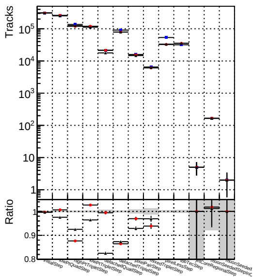
Number of tracks vs collection DQMstep3_SoftQCD_CKF DQMstep3_SoftQCD_default DQMstep3_SoftQCD_defaultNEWT2
