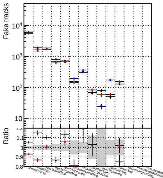
—●— DQMstep3_SoftQCD_CKF —●— DQMstep3_SoftQCD_default —●— DQMstep3_SoftQCD_defaultNEWT2
