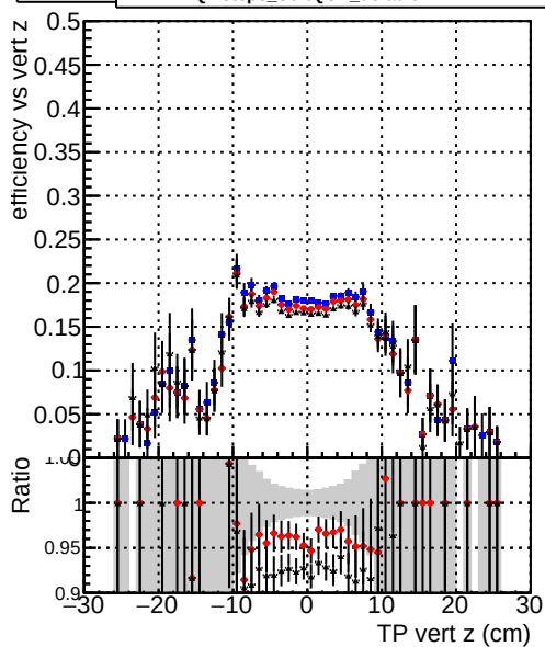
Efficiency vs vert z —●— DQMstep3_SoftQCD_CKF —●— DQMstep3_SoftQCD_default —●— DQMstep3_SoftQCD_defaultNEWT2
