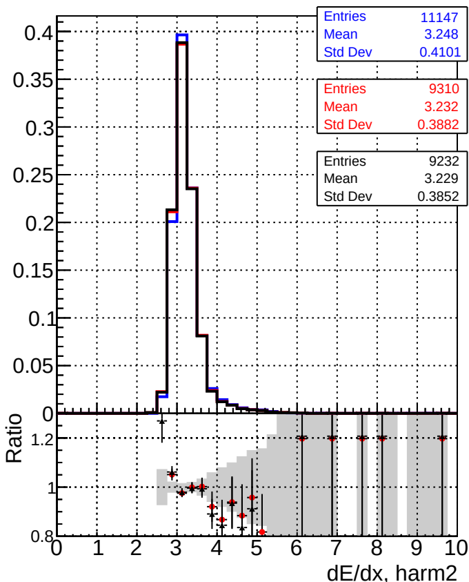
— DQMstep3_SoftQCD_CKF — DQMstep3_SoftQCD_default — DQMstep3_SoftQCD_defaultNEWT2
