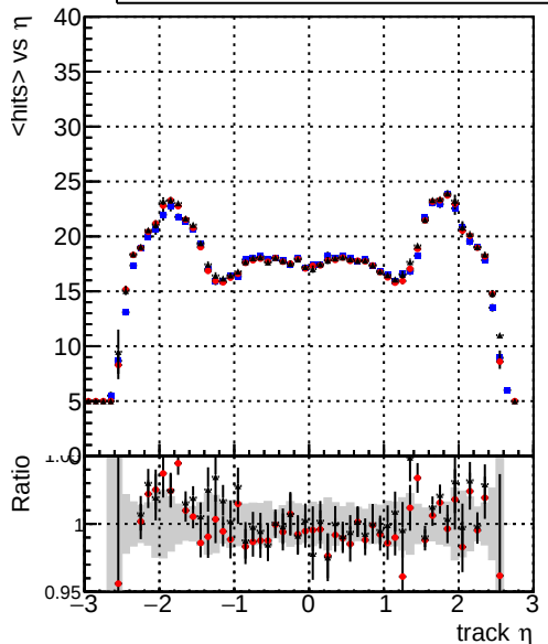
— DQMstep3_SoftQCD_CKF — DQMstep3_SoftQCD_default — DQMstep3_SoftQCD_defaultNEWT2 mean hits
