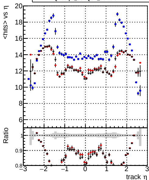
— DQMstep3_SoftQCD_CKF — DQMstep3_SoftQCD_default — DQMstep3_SoftQCD_defaultNEWT2 mean hit
