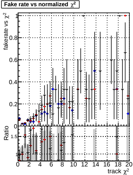
Fake rate vs. DOMstep3 SoftOCD-CKF SoftOCD-default DOMstep3 SoftOCD-default NEWT2
