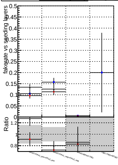
Fake rate vs. DOMstep3 SoftOCD-CKF SoftOCD-default DOMstep3 SoftOCD-default NEWT2
