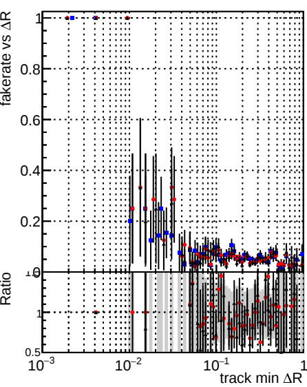
Legend: DQMstep3_SoftQCD_CKF (blue squares), DQMstep3_SoftQCD_default (red circles), DQMstep3_SoftQCD_defaultNEWT2 (black line)
