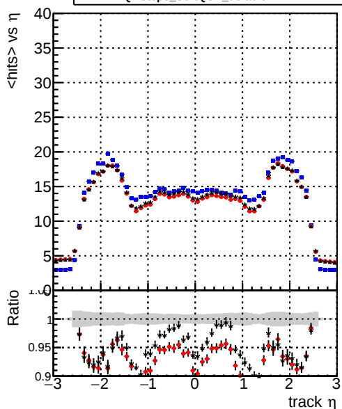
— DQMstep3_SoftQCD_CKF — DQMstep3_SoftQCD_default — DQMstep3_SoftQCD_defaultNEWT2
