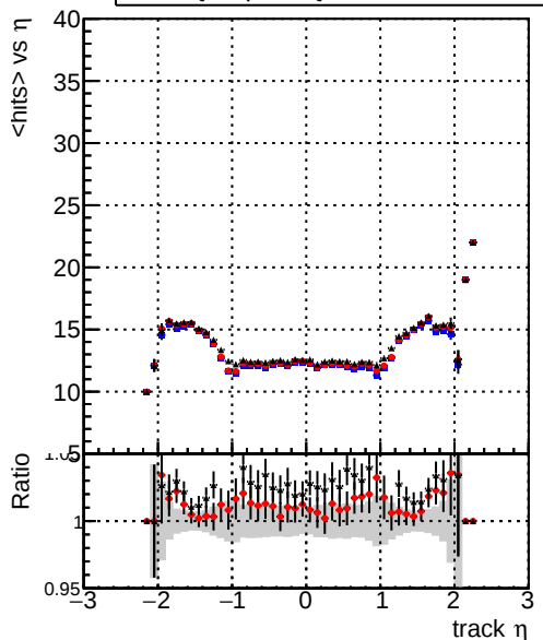
DQMstep3_SoftQCD_CKF DQMstep3_SoftQCD_default DQMstep3_SoftQCD_defaultNEWT3 mean hits
