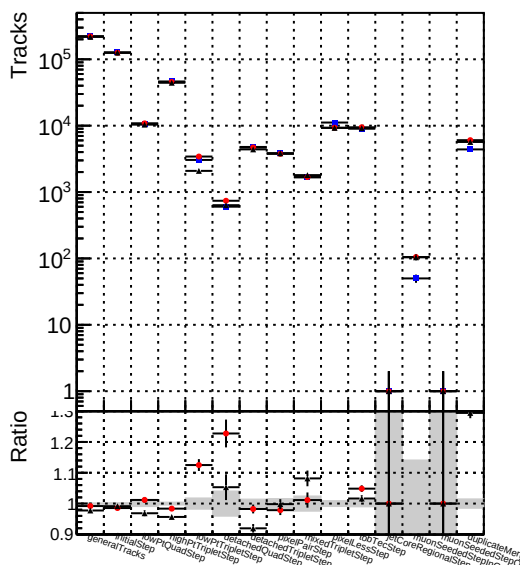
—●— DQMstep3_SoftQCD_CKF —●— DQMstep3_SoftQCD_default —●— DQMstep3_SoftQCD_defaultNEWT3
