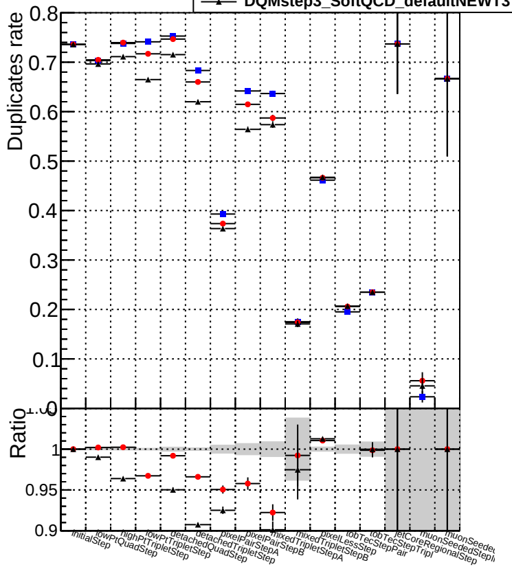
Duplicates rate vs \epsilon —●— DQMstep3_SoftQCD_default —▲— DQMstep3_SoftQCD_defaultNEWT3
